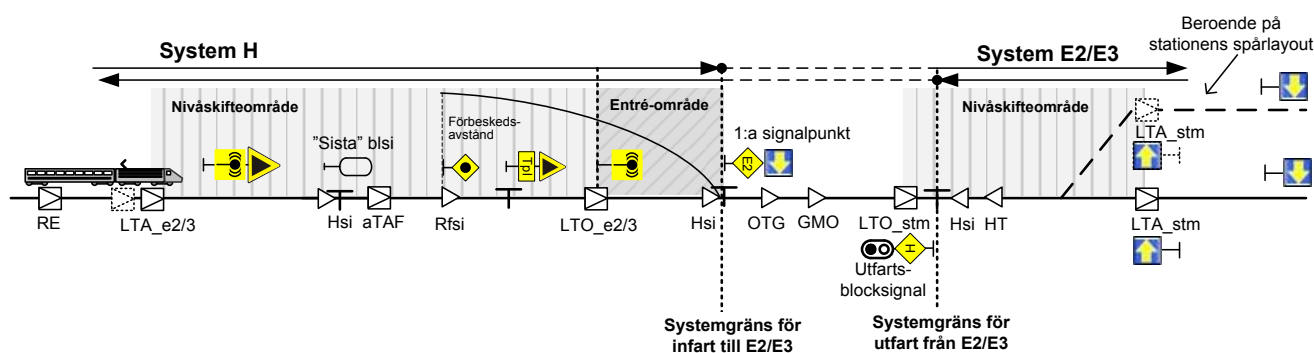
Figur 3; Gräns mot System H (linje) – Alternativ 2a, villkor för hinderfrihet i entré-området kontrolleras av RBC/IL
