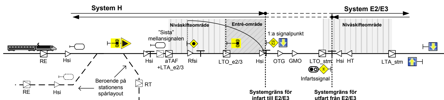
Figur 7; Gräns mot system H (driftplats) – Alternativ 2
