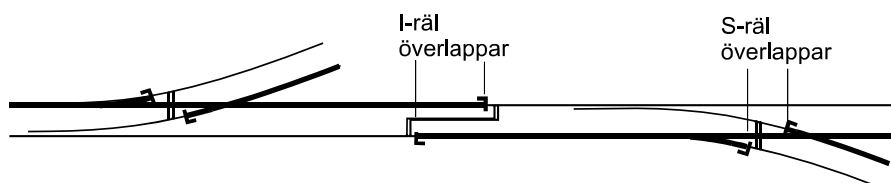
figur 13 Förskjutning i längdled av motstående isolerskarvar
