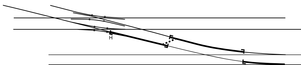
figur 21 Avgränsningar vid en dubbel korsningsväxel med skyddsväxelfunktion
