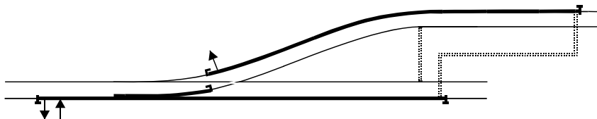
figur 8 Princip för längdmätning av växelspårledning
