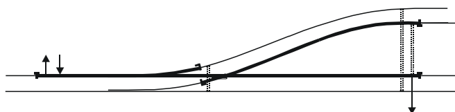
figur 16 Parallellkopplad I-räl
