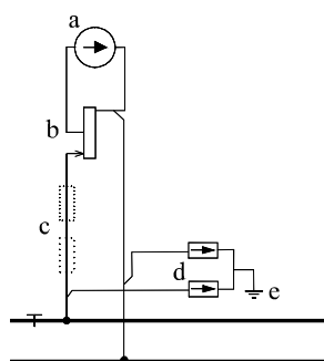
figur 7 Spårledningsupptag med åsköverspänningsskydd
