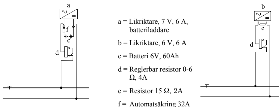
figur 6 Spårledningsmatning med respektive utan batteri
