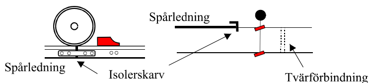
figur 2 Avgränsning vid en lokalmanövrerad spårspärr
