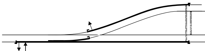
figur 15 Seriekopplad I-räl
