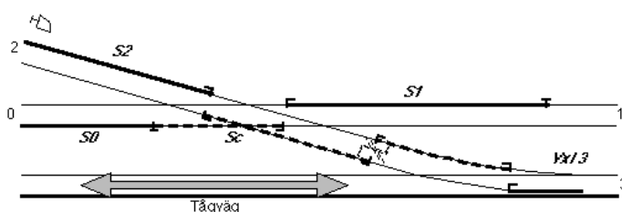
figur 22 Spårkorsning med en gemensam spårledning Sc.
