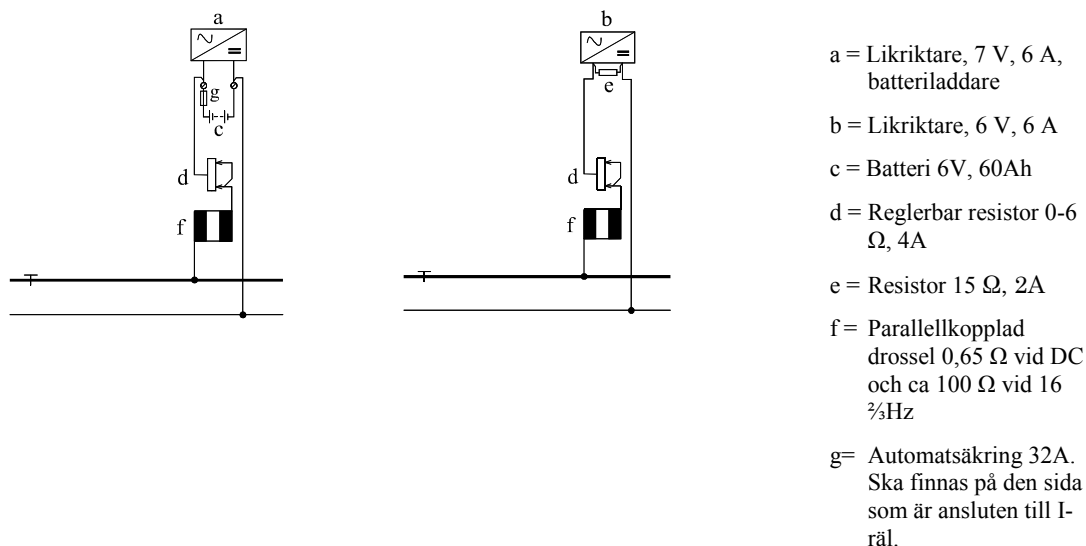
figur 4 Spårledningsmatning med respektive utan batteri
